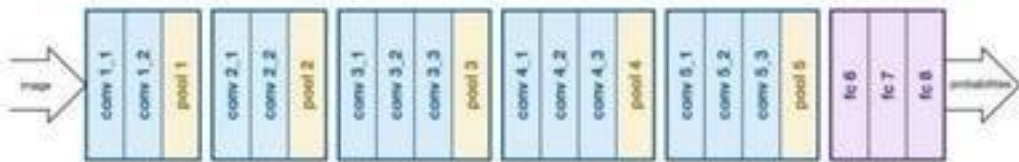
VGG-16
